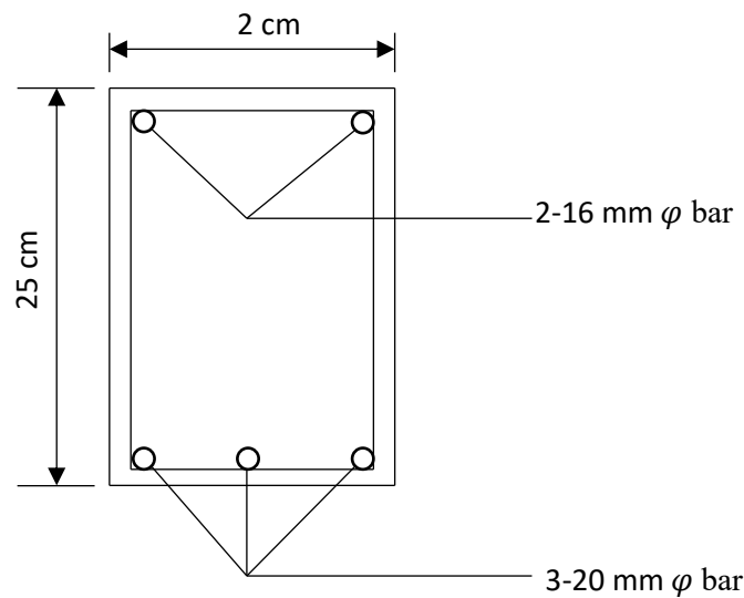
চিত্র : আয়তাকার বিম সেকশন
